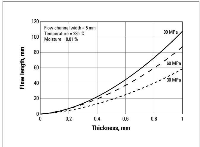
Fig. a.52 RYNITE® 555 NC010
