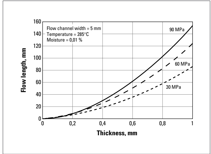
Fig. a.50 RYNITE® 530 NC010
