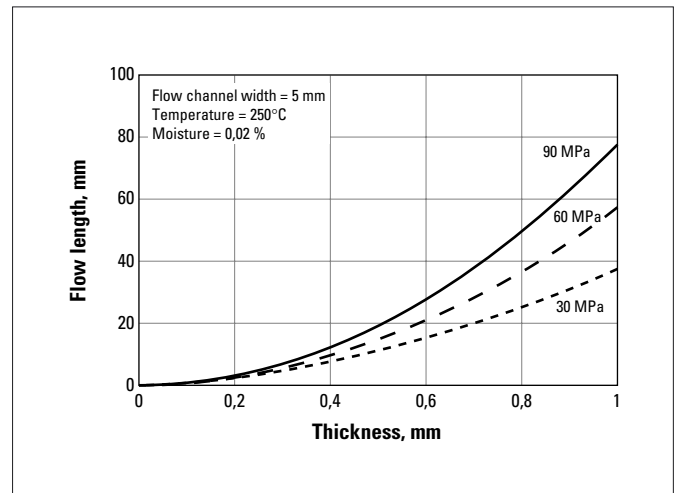
Fig. a.22 CRASTIN® ST820 NC010
