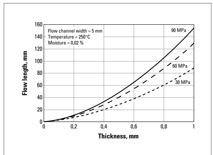
Fig. a.24 CRASTIN® T803 NC010
