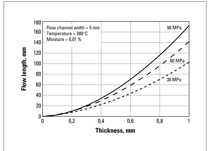
Fig. a.58 RYNITE® FR530L NC010
