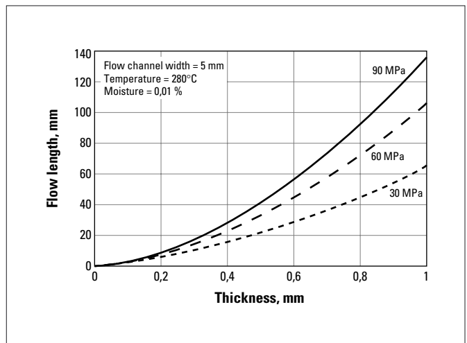
Fig. a.54 RYNITE® 940 BK505
