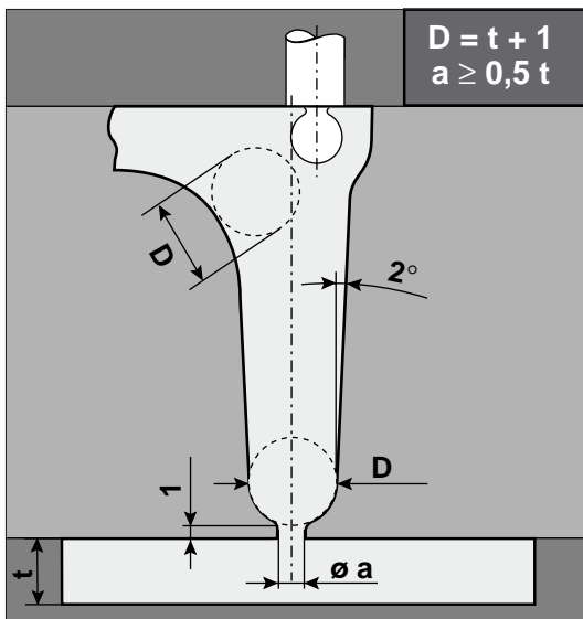
Fig. 4.7 3-Plate gate
