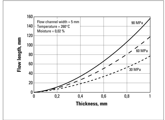
Fig. a.44 CRASTIN® LW9330FR NC010
