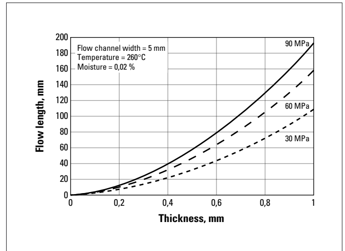
Fig. a.20 CRASTIN® SK9220 NC010
