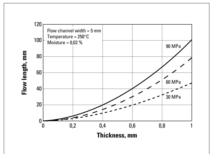
Fig. a.36 CRASTIN® SK645FRC NC010
