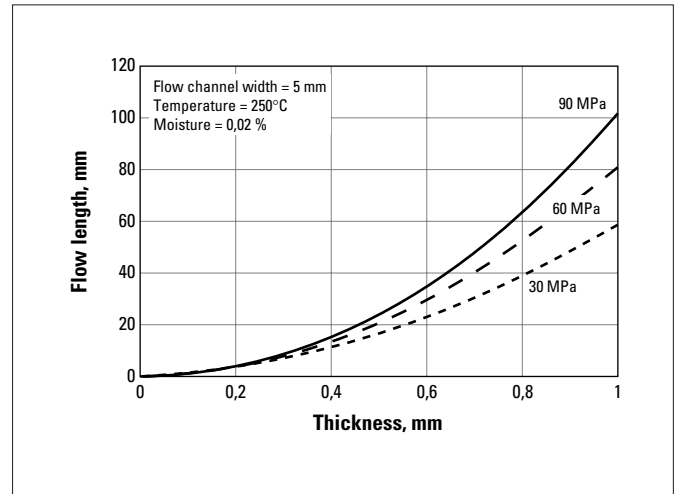
Fig. a.46 CRASTIN® SK655FR1 NC010
